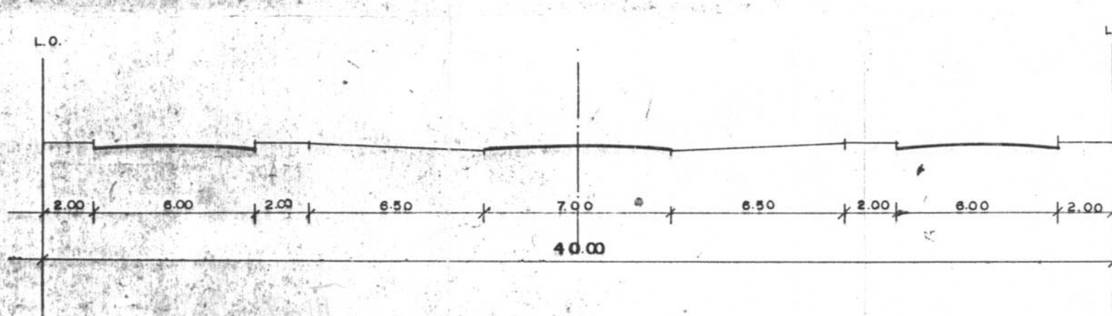
PERFIL C'-C
