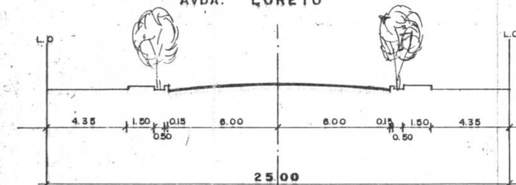
PERFIL C'-C
