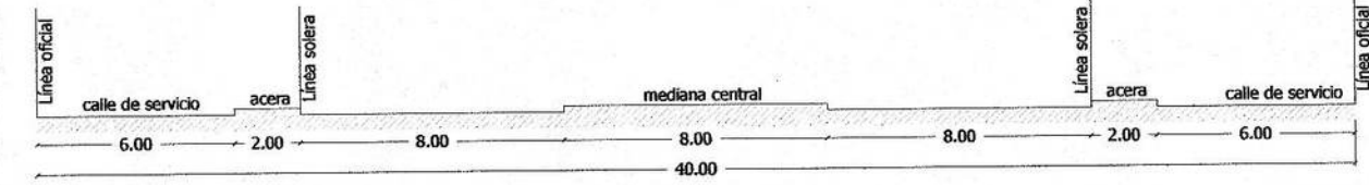
Perfil tipo Av. Longitudinal
