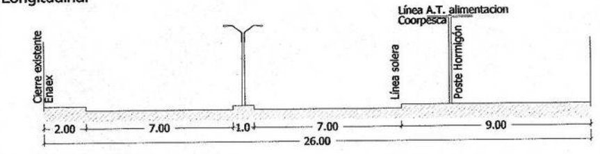
Perfil tipo Av. Segunda Industrial
